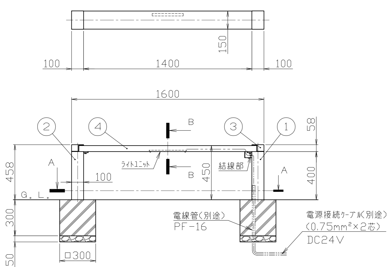
施工位置寸法(A-A断面図)
