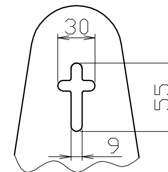
取付孔詳細図 S = 1 / 3
