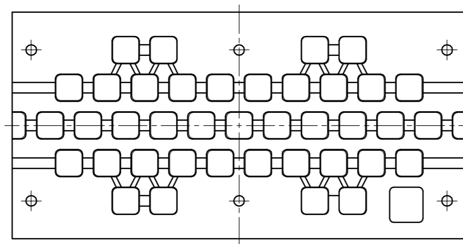
底面 (A 矢視図)
