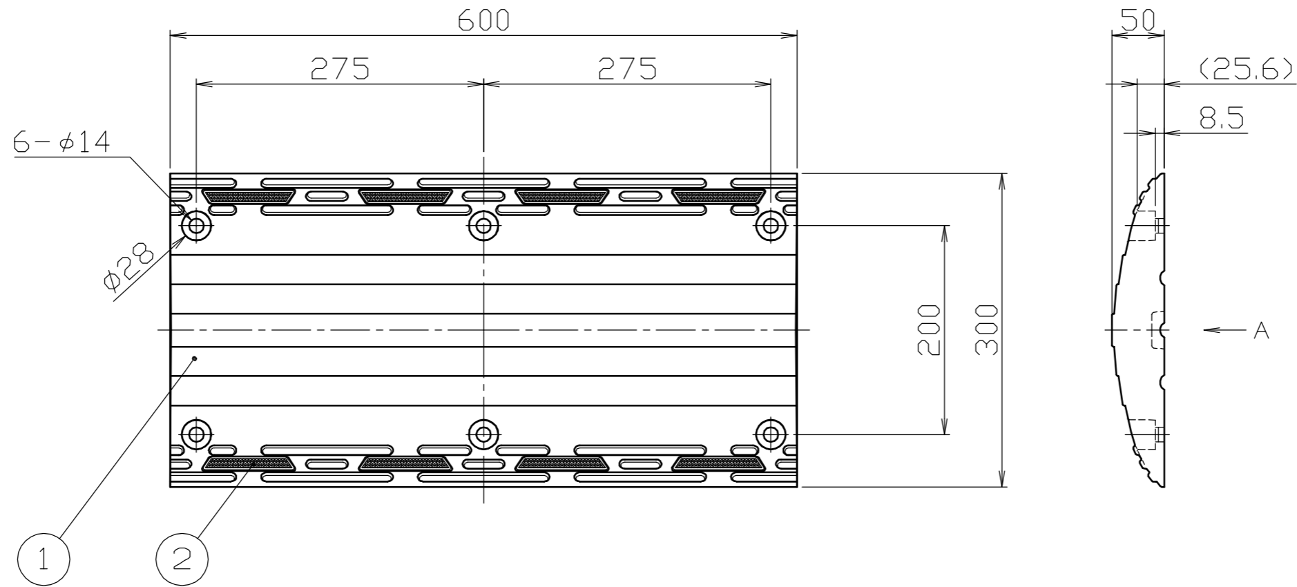
底面 (A 矢視図)
