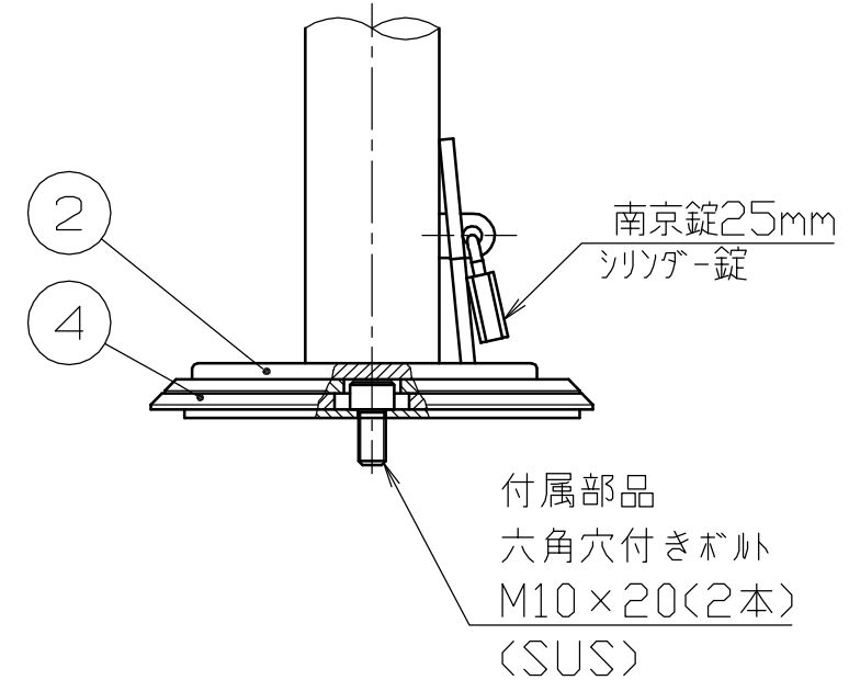
施錠部詳細図 S = 1 / 3
