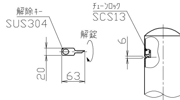
頭部詳細図 S = 1 / 5
