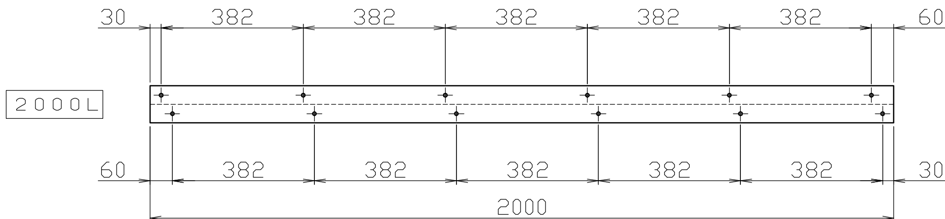
ビス穴ピッチ図 S = 1 / 10
