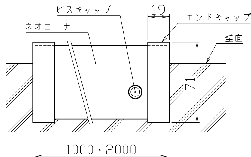
立面図
