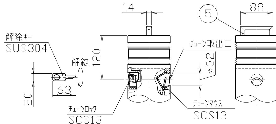
頭部取手詳細図 S = 1 / 5
