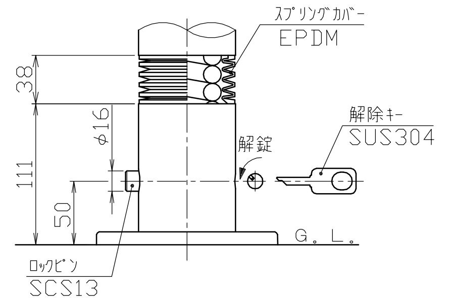
地際部・スプリング部詳細図
