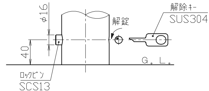
地際部詳細図 S = 1 / 3
