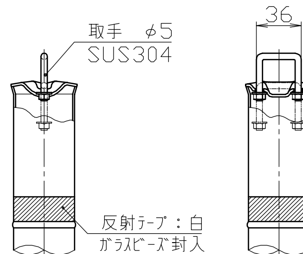
頭部取手詳細図 S = 1 / 3
