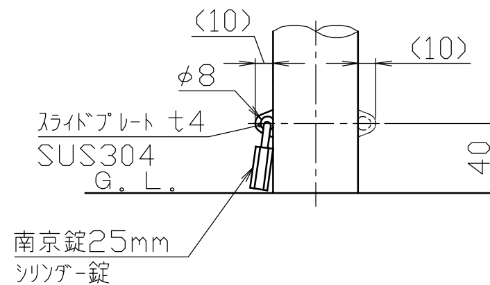
地際部詳細図 S = 1 / 3
