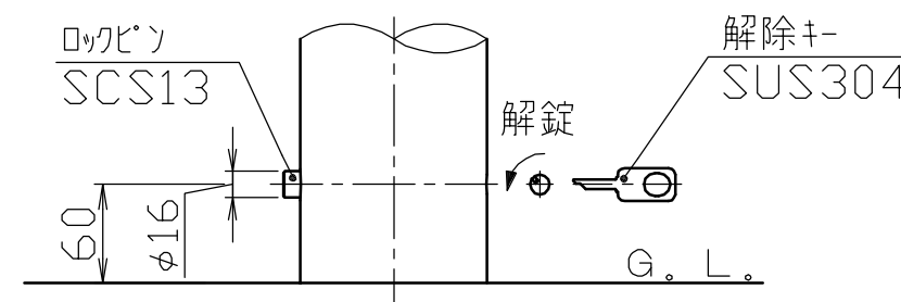
地際部詳細図 S = 1 / 5
