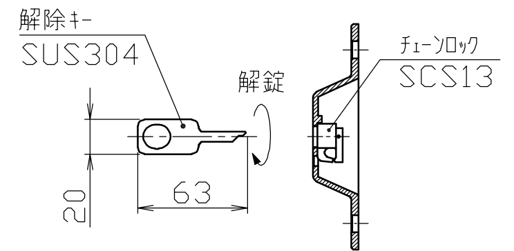
頭部ロック詳細図 S = 1 / 3
