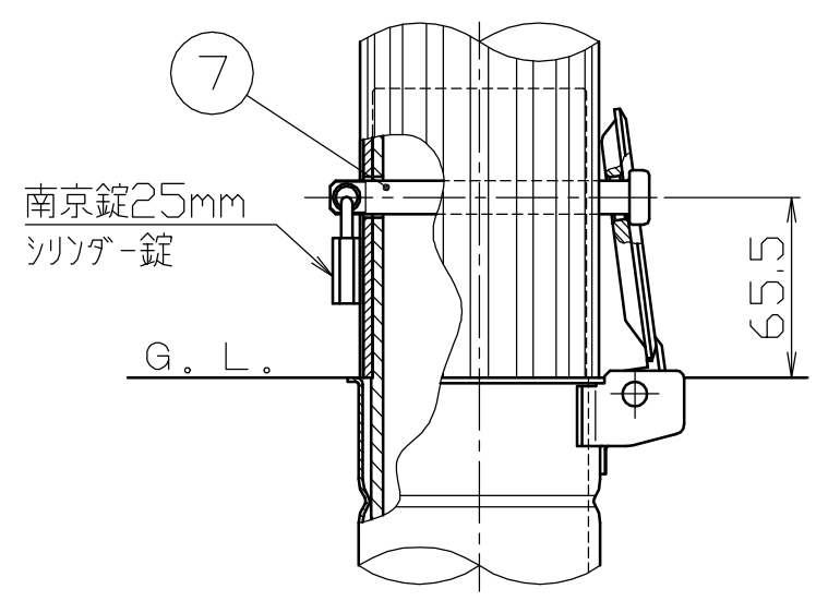
施錠部詳細図 S = 1 / 3
