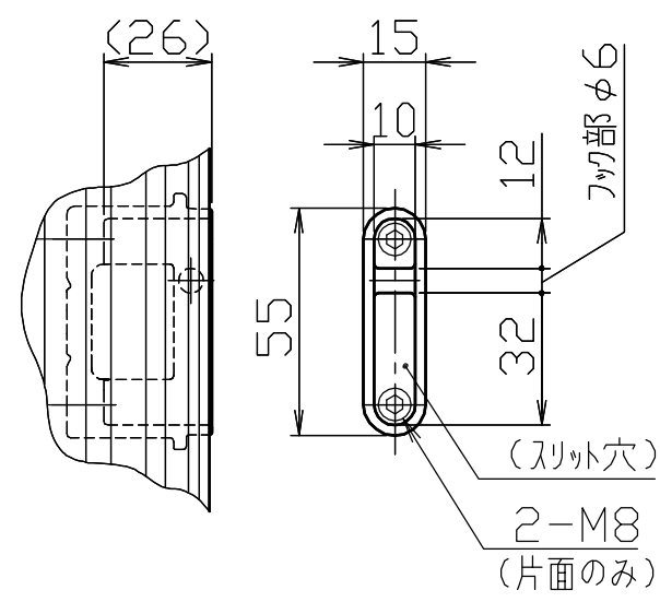
施錠部詳細図 S = 1 / 3
