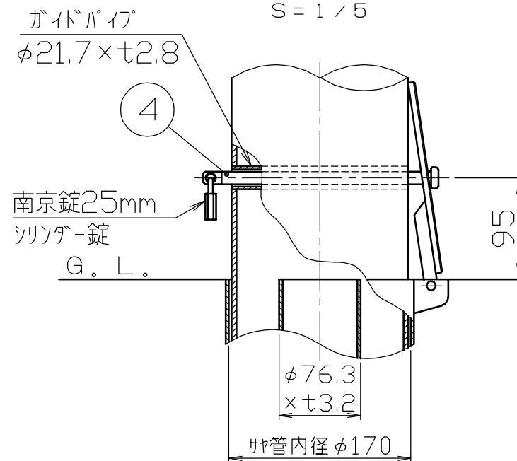
施錠部詳細図 S = 1 / 5
