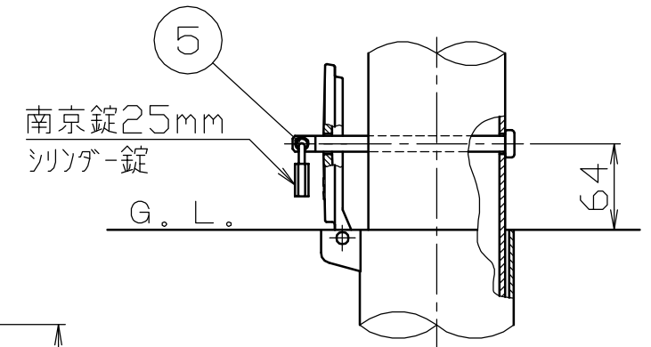
施錠部詳細図 S = 1 / 5
