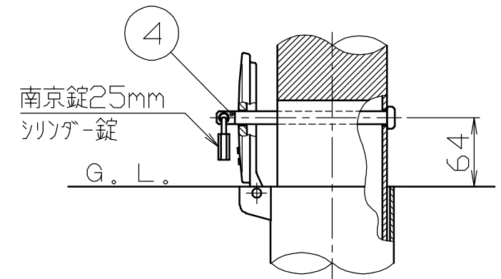
施錠部詳細図 S = 1 / 5
