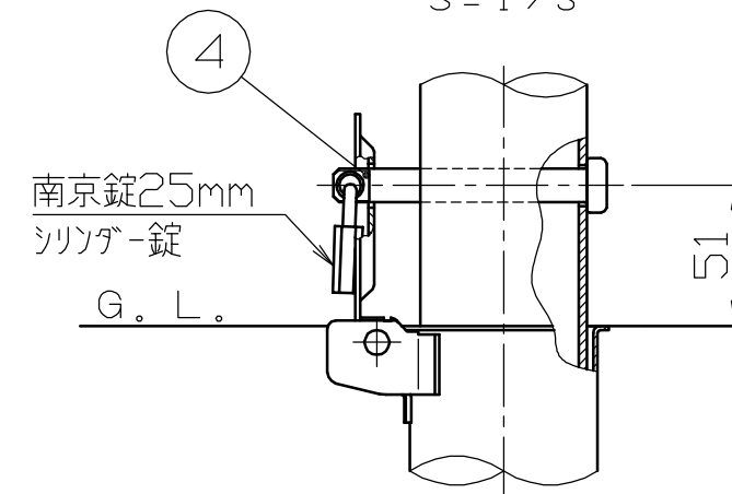
施錠部詳細図
