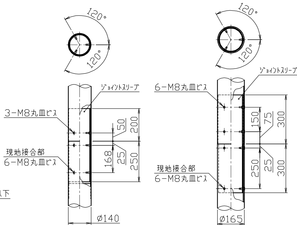
ジョイント部詳細図 S=1/10
