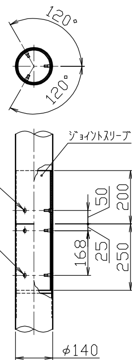
ジョイント部詳細図 S=1/10
