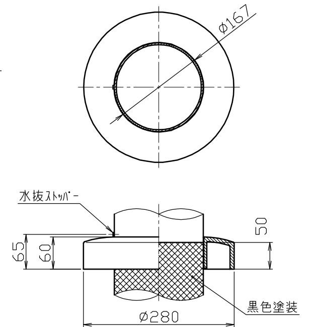
グラウンドセット詳細図 S=1/5
