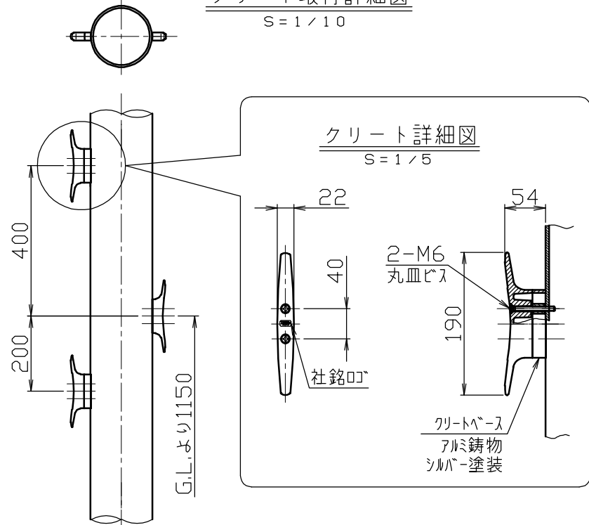
クリーン取付詳細図
