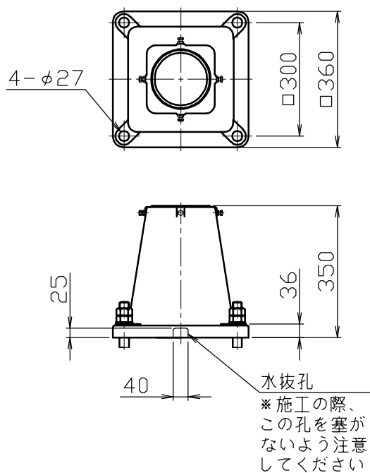
ベース詳細図
