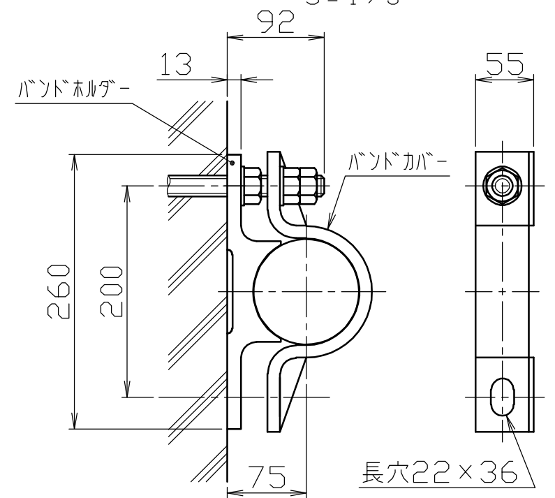
バンド詳細図 S = 1 / 5
