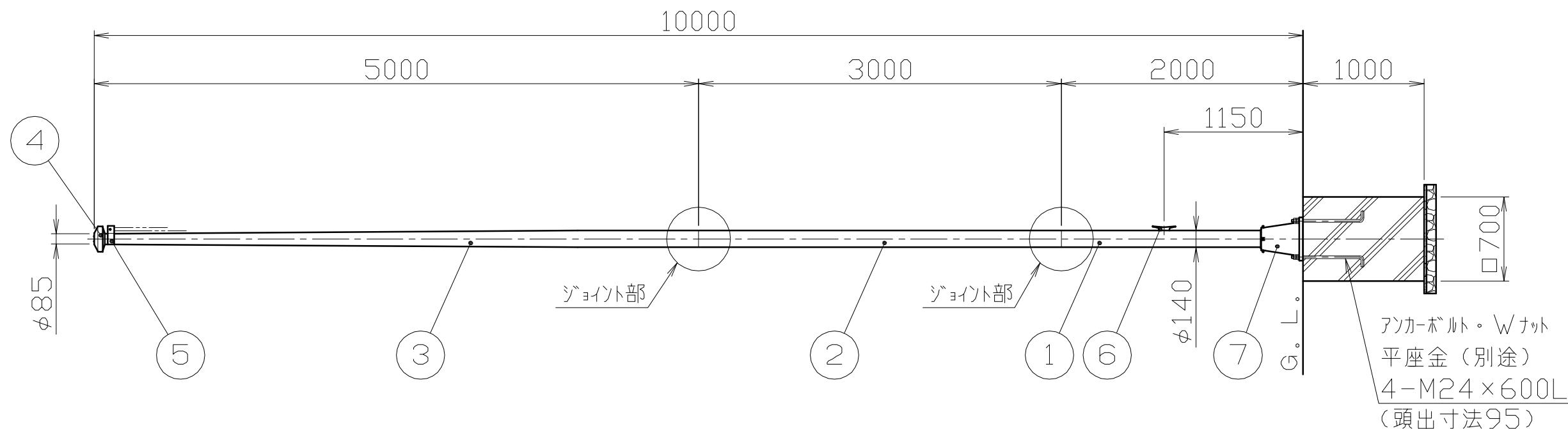
冠頭部詳細図 S = 1 / 10
