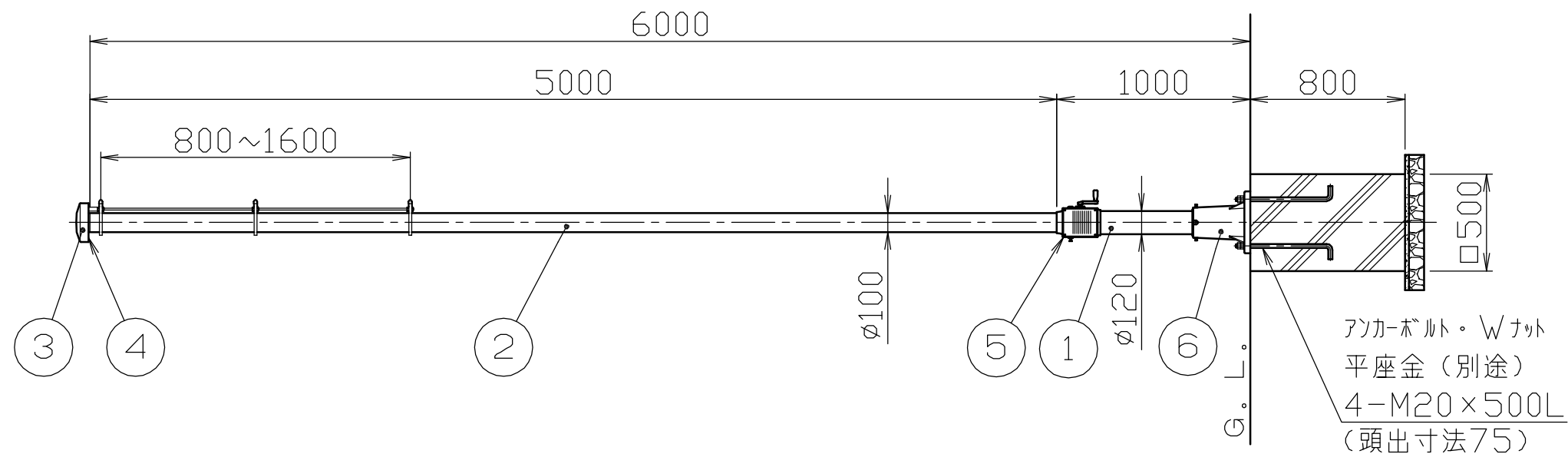
冠頭部詳細図 S = 1 / 10
