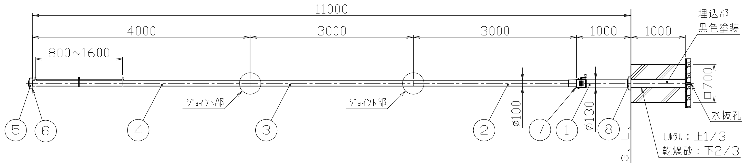
冠頭部詳細図 S = 1 / 1 0
