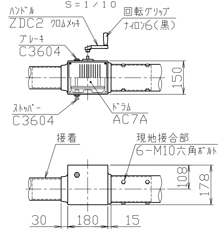
ハンドル部詳細図
