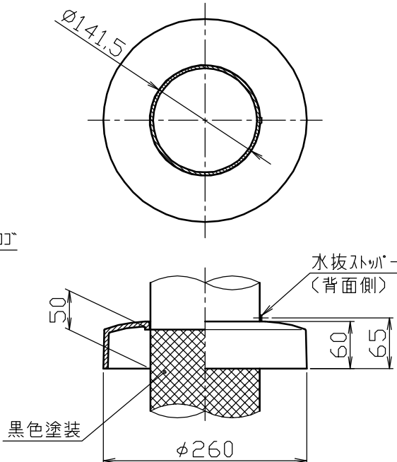
グラウンドセット詳細図 S=1/5
