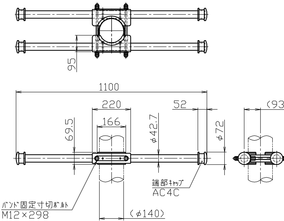
バナー下固定部詳細図
