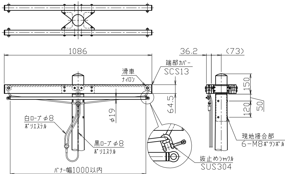
頭部横バ-詳細図
