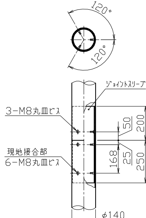
ジョイント部詳細図
