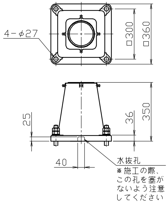
ベース詳細図
