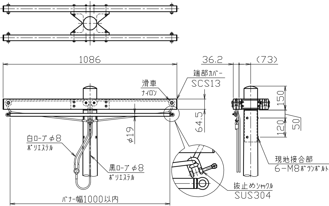
バナー下固定部詳細図
