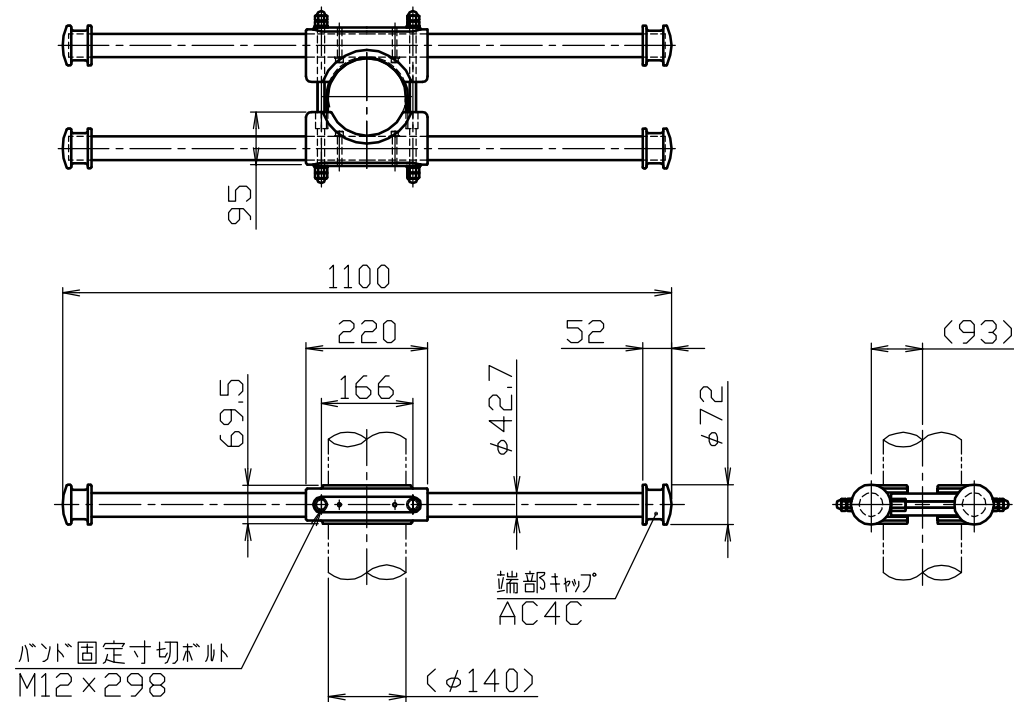
バナー下固定部詳細図
