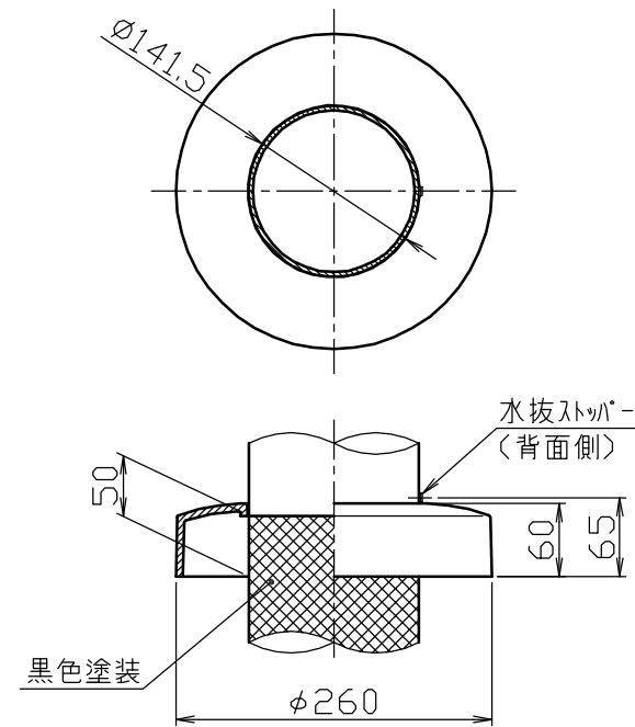
グランドセット詳細図 S=1/5
