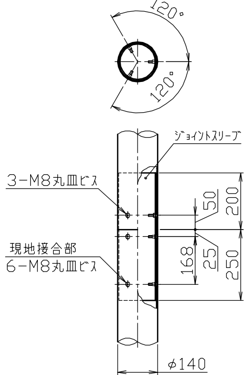
ベース詳細図 S=1/10
