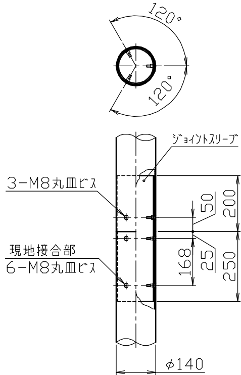
グラウンドセット詳細図 S=1/5
