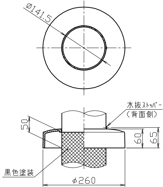
グラウンドセット詳細図 S=1/5
